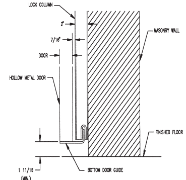
DETAIL D - BOTTOM DOOR GUIDE SECTION
